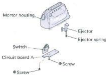
قطعات بدنه، بالابنده، کلید و صفحه اتصال
